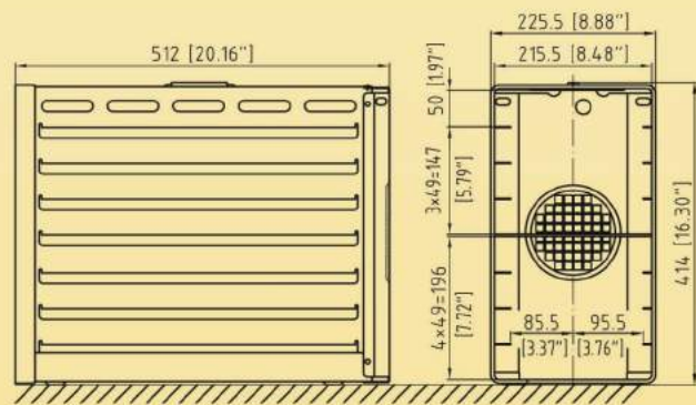
P/N: R80004-A01
