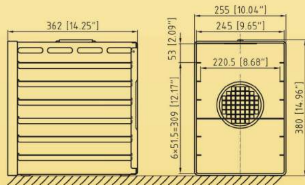
P/N: R70005-K01
