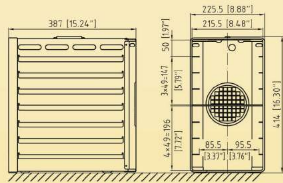
P/N: R80001-A01
