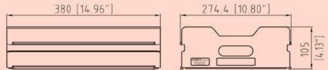
P/N: DS0003-A01
